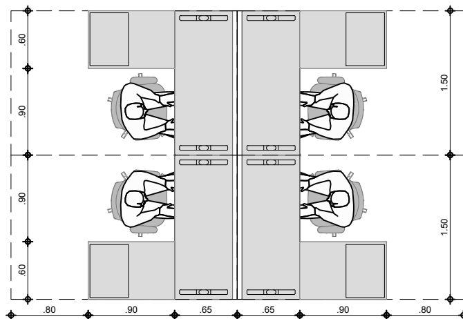
ARQUITECTURA EMPRESARIAL
