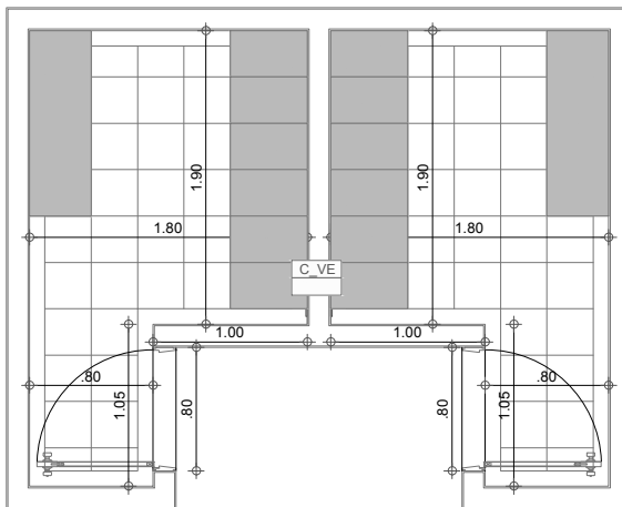
VESTIER 8.95 m 2
